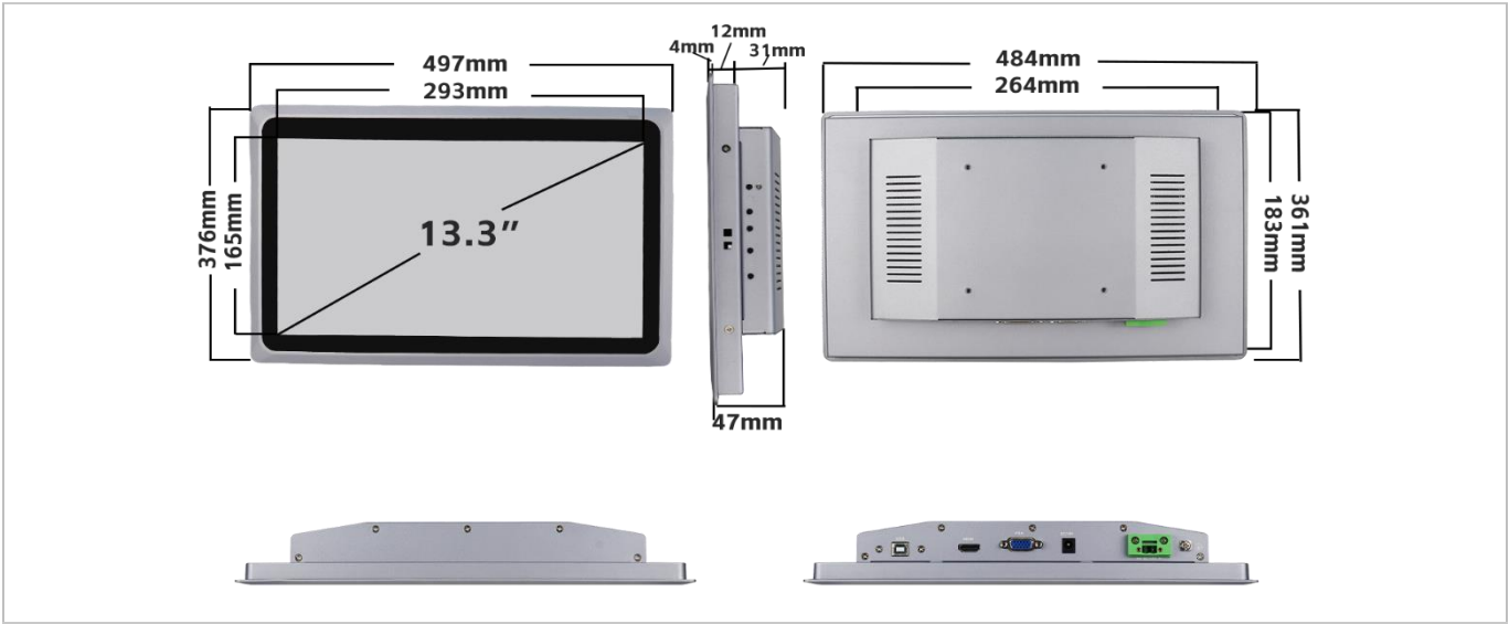
产品尺寸
