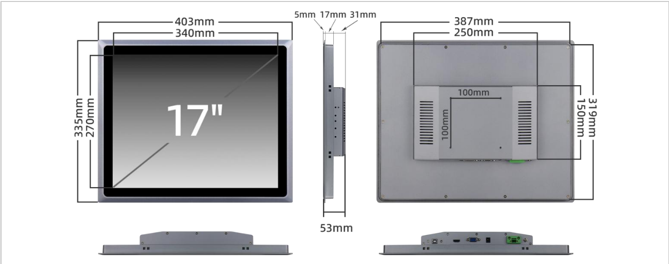
产品尺寸
